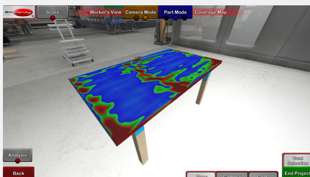
Vérification de l'application de la bonne épaisseur de peinture
